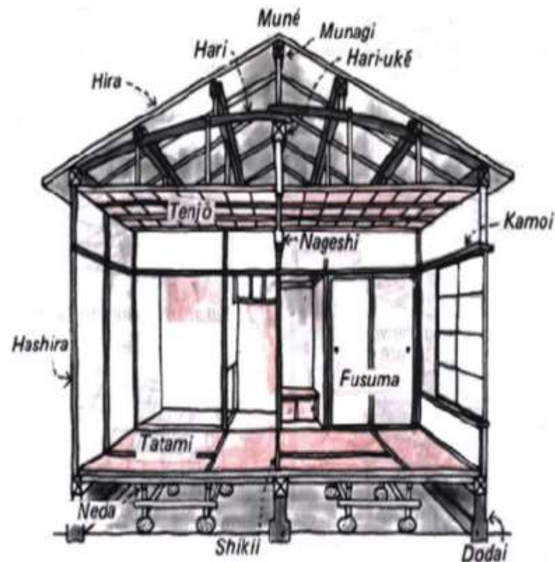
Cotruzione di una piccola casa nello stile tradizionale
